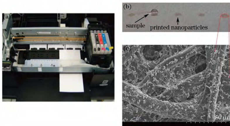
图 2 (a)制作 SERS 基底所用的喷墨打印机;(b)在纳米颗粒区域沾有样品的喷墨打印法打印所得的试纸; (c)试纸表面的 Ag NPs 的扫描电镜图 [31]
